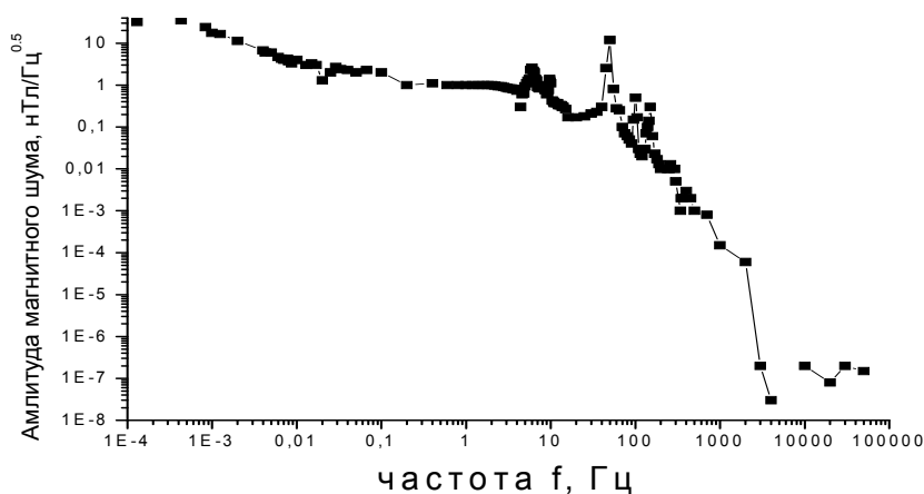
Рис.4. Зависимость амплитуды спектральной плотности магнитного шума от частоты внутри экрана.
