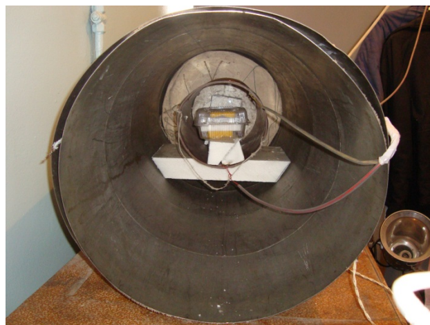
Рис.3. Внешний вид внутренней части установки.
