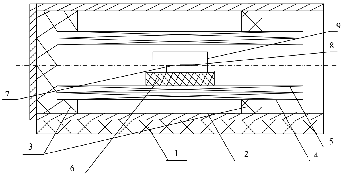
Рис.1. Вид экспериментальной установки в разрезе. 1 – демпфирующая резина; 2 – двухслойный пермалловый экран с дном.; 3 – кольца из немагнитного материала, центрирующие обмотки соленоида относительно центральной оси экрана; 4 и 5 – обмотки соленоида; 6 – подставка из немагнитного материала; 9 – влажная камера; 7 – подставка из немагнитного материала внутри влажной камеры; 8 – корни кресс-салата или кукурузы.
